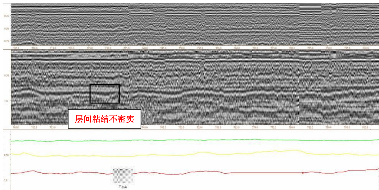
图 4.4.2-8 京沪高速 K74+605~K74+700 雷达图
