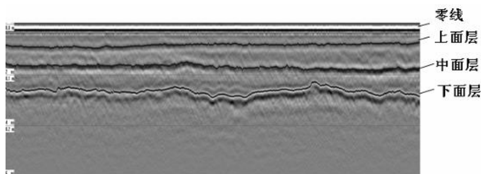
图 4.2.1-3 面层雷达检测层面追踪
