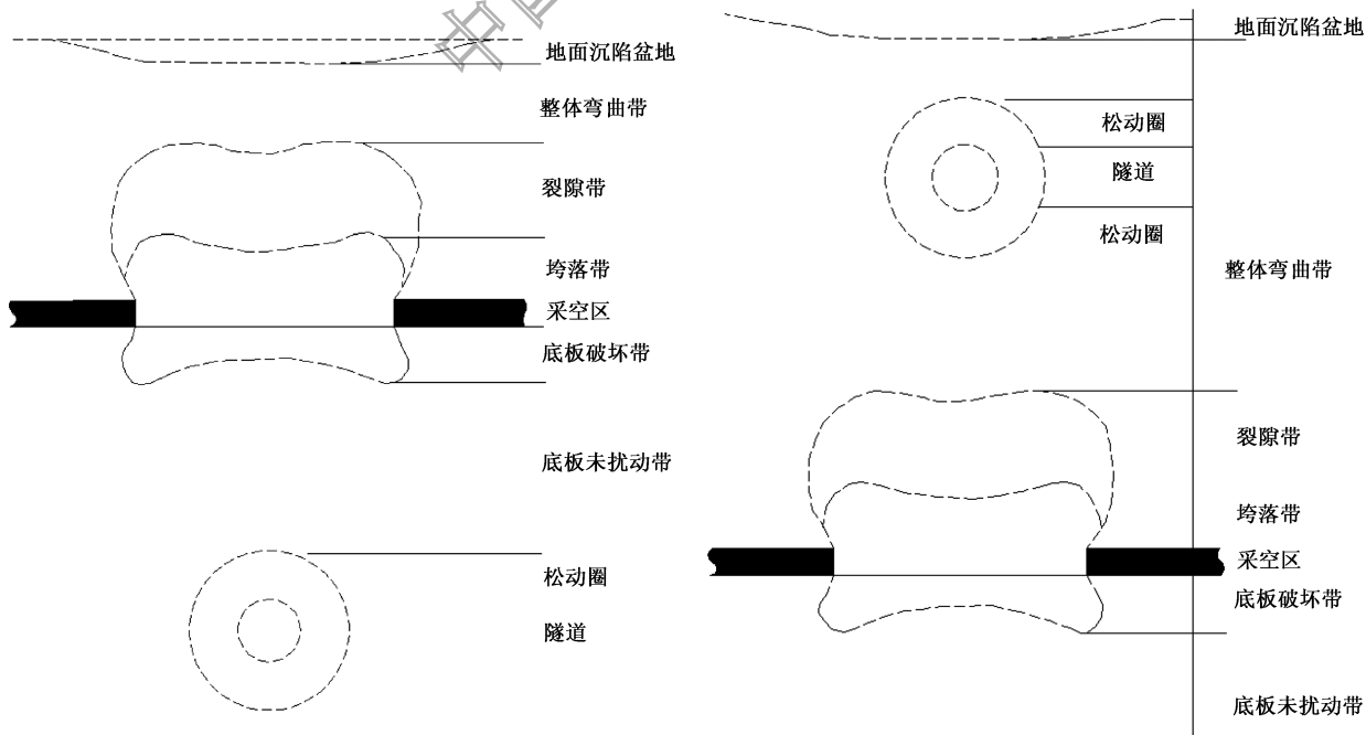
图 I.1 采空区位于隧道上方评价示意图
