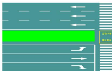
图4 单线式交叉口禁止行人驻足区设置示意
