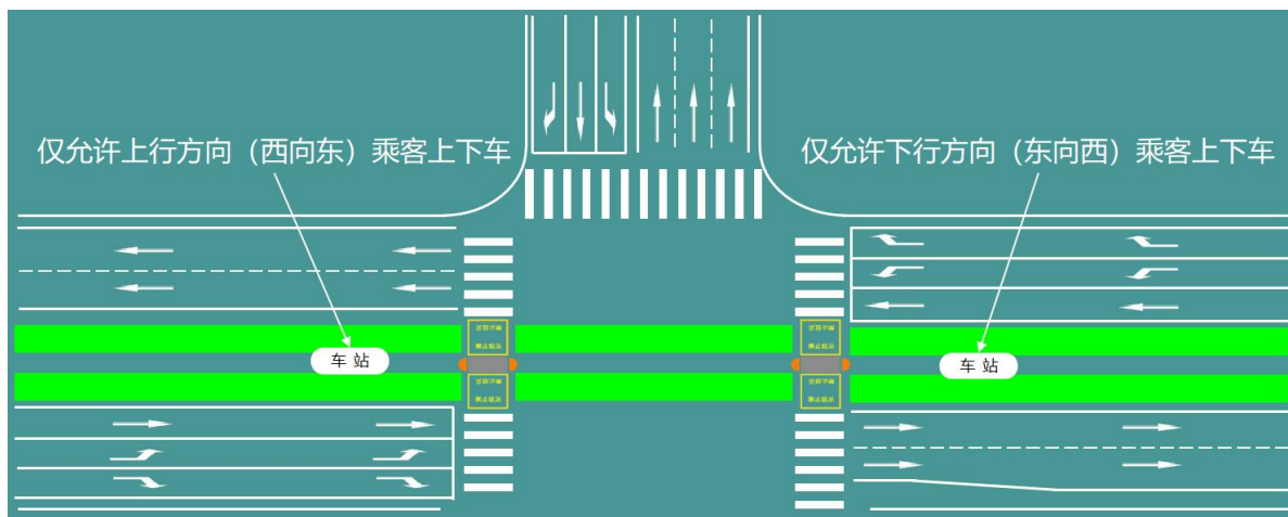
图 10 错位岛式车站示意
