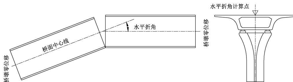
图 18 梁端水平折角示意图
